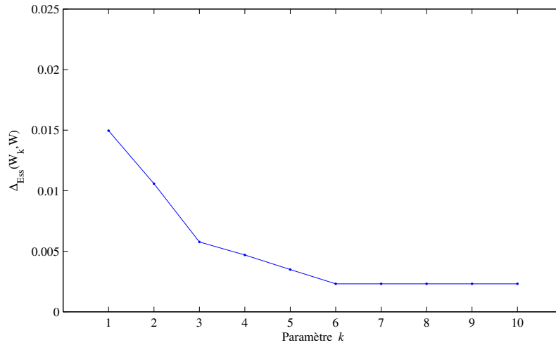
Figure 4.2 – Différence d'utilisation des gènes essentiels intervenant dans k\text{-SIP}_{col} et \mathcal{G}_{col} en fonction de k . L'étude différentielle est réalisée en utilisant la formule \Delta_{Ess}(W_k, W) , avec W_k l'ensemble des gènes intervenant dans les k\text{-SIPs} de k\text{-SIP}_{col} et W l'ensemble des gènes intégrés à \mathcal{G}_{col} .
