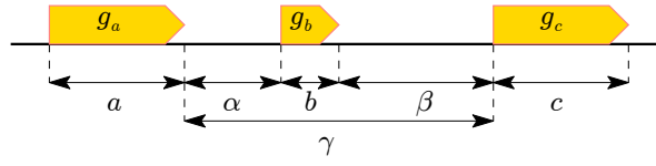
Figure 3.8 – Exemple de distance intergénique sur un chromosome. Les gènes g_a , g_b et g_c sont composés respectivement de a , b et c nucléotides. La distance intergénique entre g_a et g_b est de \alpha nucléotides, celle entre g_b et g_c est de \beta nucléotides, et celle entre g_a et g_c est de \gamma = \alpha + b + \beta nucléotide. Cet exemple montre que la distance intergénique ne respecte pas l'inégalité triangulaire, car \alpha + \beta < \gamma .
