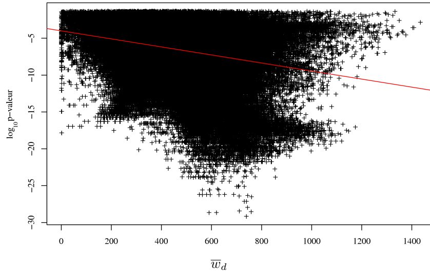
Figure 4.1 – Nuage de points présentant les 1-SIPs de 1-SIP_{col} sous la formes de couples (\overline{w}_d, p\text{-valeur}) . Chaque point représente un 1-SIP. La droite rouge est la droite de régression linéaire du nuage de points. Son R^2 est de 0,074
