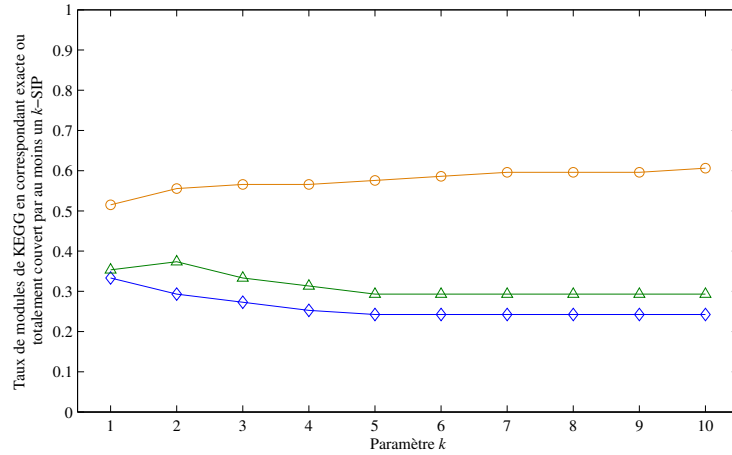
Figure 4.7 – Intérêt modulaire de tous les k -SIPs de k\text{-SIP}_{col} pour des k distincts dans E. coli . La courbe \circ représente les taux de modules de KEGG qui sont couverts totalement par au moins un k -SIP. Le courbe \diamond (la courbe \triangle respectivement) résume le taux de modules seul (ou en couple respectivement) qui correspondent exactement à des k -SIPs.
