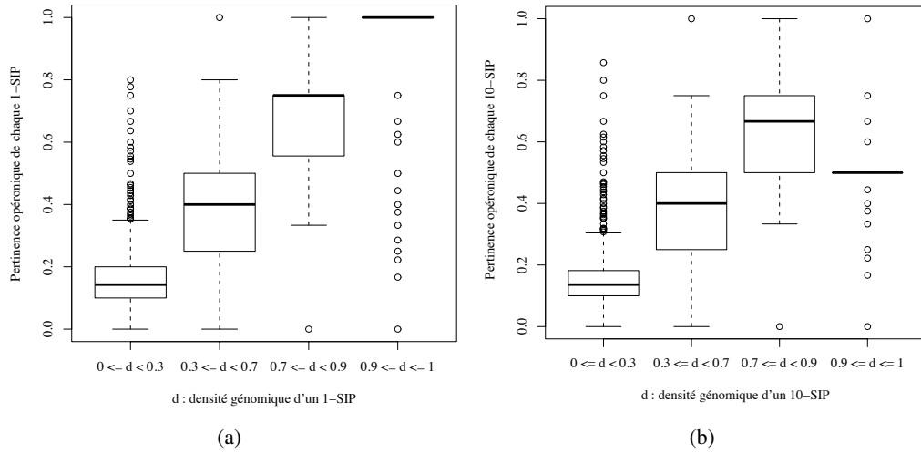
Figure 4.5 – Taux de correspondance, pour k = 1 et 10, entre les k -SIPs de k - SIP_{col} regroupés par densité génomique et les opérons d’ E. coli en utilisant la mesure de Jaccard. Pour chaque k -SIP sip , la densité génomique d_G(sip) et la pertinence opéronique P_o = \max_{op \in Opéron} \{Jaccard(sip, op)\} donnent les abscisses et ordonnées d’un point dans le graphe. Les points sont regroupés en quatre classes de densité (axe des abscisses), et une boîte est dessinée dans chacune de ces classes afin de résumer, pour les k -SIPs de la classe donnée, le score P_o (axe des ordonnées). Les limites supérieures et inférieures d’une boîte sont les valeurs des 1 er et 3 e quartiles de la classe qu’elle résume, et chaque extension au delà des limites de la boîte couvre les k -SIPs qui ne sont pas plus distant de 1,5 fois la hauteur de la boîte. Les points en dehors de ces extensions correspondent aux k -SIPs qui se différencient trop de ceux dans la boîte.
