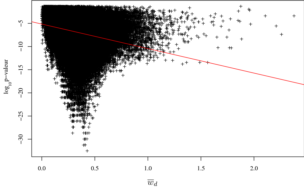
Figure 4.12 – Nuage de points présentant les 1-SIPs de 1-SIP_{coexp} sous la formes de couples (\bar{w}_d, \text{p-valeur}) . Chaque point représente un 1-SIP. La droite rouge est la droite de régression linéaire du nuage de points. Son R^2 est de 0,078.
