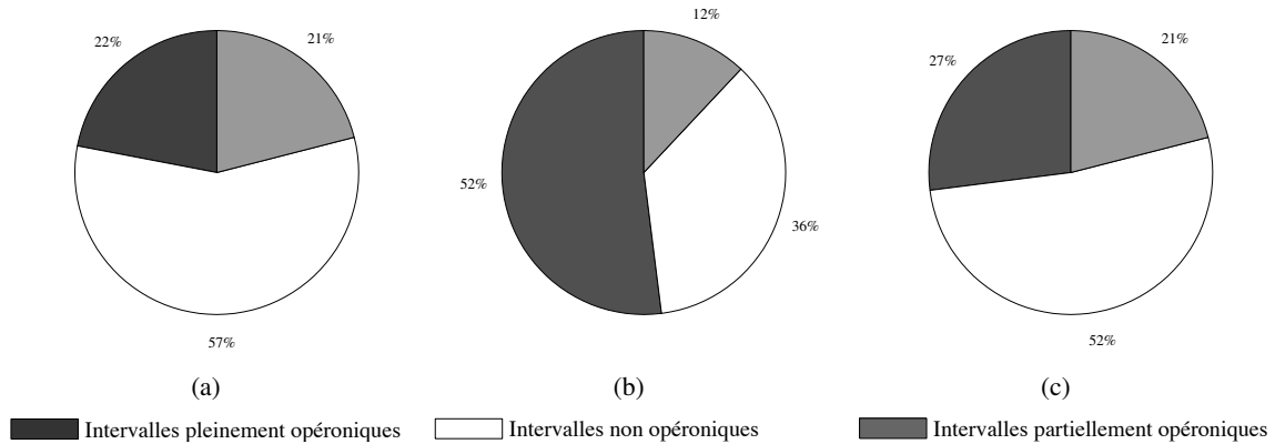
Figure 5.4 – Intérêt opérionique des intervalles communs. Proportion d’intervalles communs qui sont (1) pleinement opérioniques (FOI), (2) non opérioniques (NOI), et (3) partiellement opérioniques (FOI) pour (a) tous les intervalles communs, (b) les intervalles communs maximaux, et (c) les intervalles communs aléatoires.
