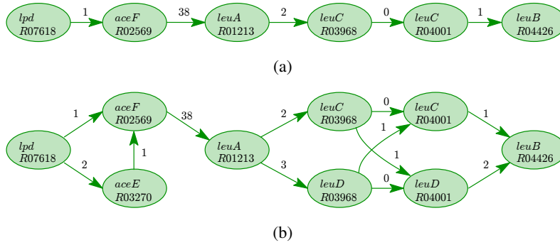
Figure 3.2 – Exemples de k -SIPs issus d' E. coli : (a) un 1-SIP ( \bar{w}_d = 7 ) et (b) un 5-SIP ( \bar{w}_d = 7.43 ) de la réaction R07618 à la réaction R04426 .
