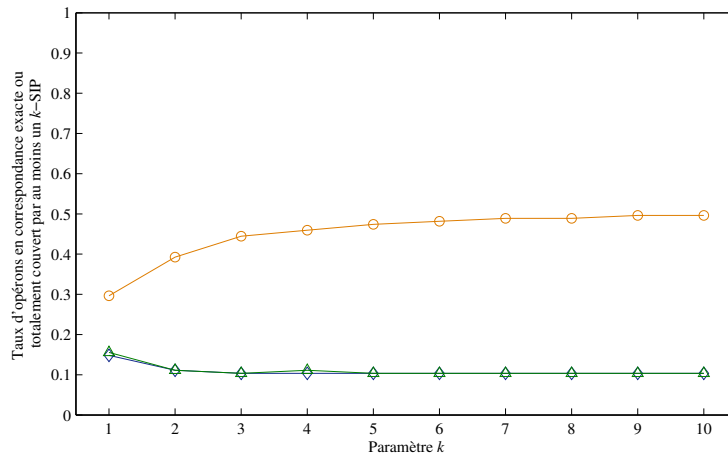
Figure 4.14 – Intérêt opéronique de tous les k -SIPs pour des valeurs de k distinctes dans E. coli . La courbe en \circ représente les taux d'opérons qui sont couverts totalement par au moins un k -SIP. La courbe en \diamond (les courbes en \triangle et en \star respectivement) présente le taux d'opérons seuls correspondant exactement à un k -SIP (le taux d'opérons seul ou en couple correspondant exactement à un k -SIP, et le taux d'opérons seuls, en couple ou en triplet correspondant exactement à un k -SIP respectivement).
