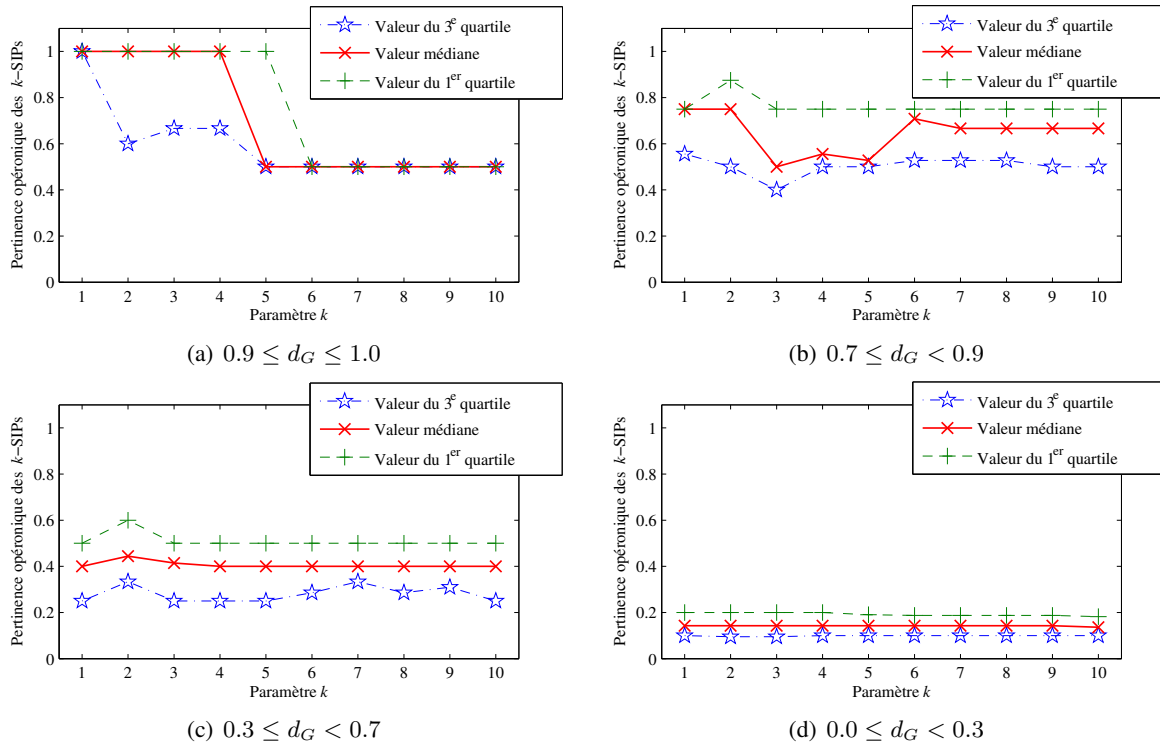
Figure 4.6 – Évolution de la pertinence opérationnelle des k -SIPs de G_{col} groupés par classe de densité génomique pour 1 \leq k \leq 10 . L'évolution de chaque classe de densité génomique : (a) 0.9 \leq d_G \leq 1.0 , (b) 0.7 \leq d_G < 0.9 , (c) 0.3 \leq d_G < 0.7 and (d) 0.0 \leq d_G < 0.3 , est résumée par trois courbes dans chaque cas : les courbes \times , + et \star représentent respectivement l'évolution de la valeur médiane, la valeur du 1 er et 3 e quartile de pertinence opérationnelle des k -SIPs de densité d .
