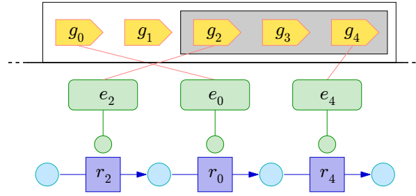
Figure 5.3 – Comparaison entre l’intervalle de gènes [g_2..g_4] donné et l’intervalle induit par un srdr -chemin allant de g_2 à g_4 . Le srdr -chemin ch allant de g_2 à g_4 est présenté ici en vue éclatée, avec les gènes (flèches épaisses) projetés sur le génome, les réactions (carrés) projetées sur le réseau métabolique formant une chaîne alternant réactions et métabolites (cercles), et les enzymes (rectangles arrondis) liant chaque gène dont elles sont le produit aux réactions qu’elles catalysent. L’intervalle de gènes [g_2..g_4] est quant à lui représenté par le cadre gris sur le génome. Nous constatons que l’intervalle de gènes [g_0..g_4] (cadre blanc) induit par ch “déborde” de [g_2..g_4] . En effet, ch utilise le gène g_0 qui n’appartient pas à [g_2..g_4] . La densité génomique de ch est d_G(ch) = \frac{3}{5} et la mesure de Jaccard entre les gènes de ch et ceux de [g_2..g_4] est égale à 0,5.
