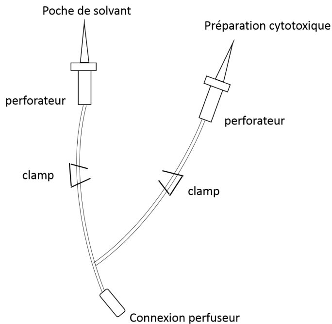
Figure 3 : Système monobras permettant l’administration sécurisée des anticancéreux
