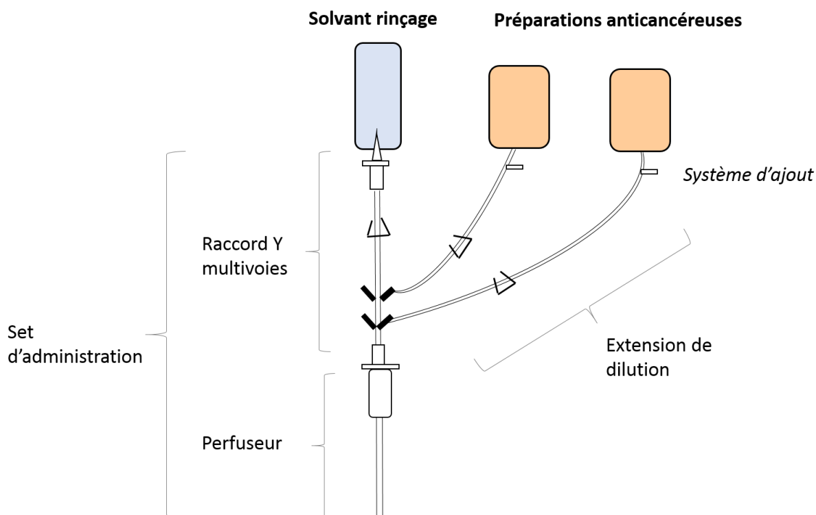
Figure 4 : Arbre à perfusion multiple permettant l'administration sécurisée des anticancéreux
