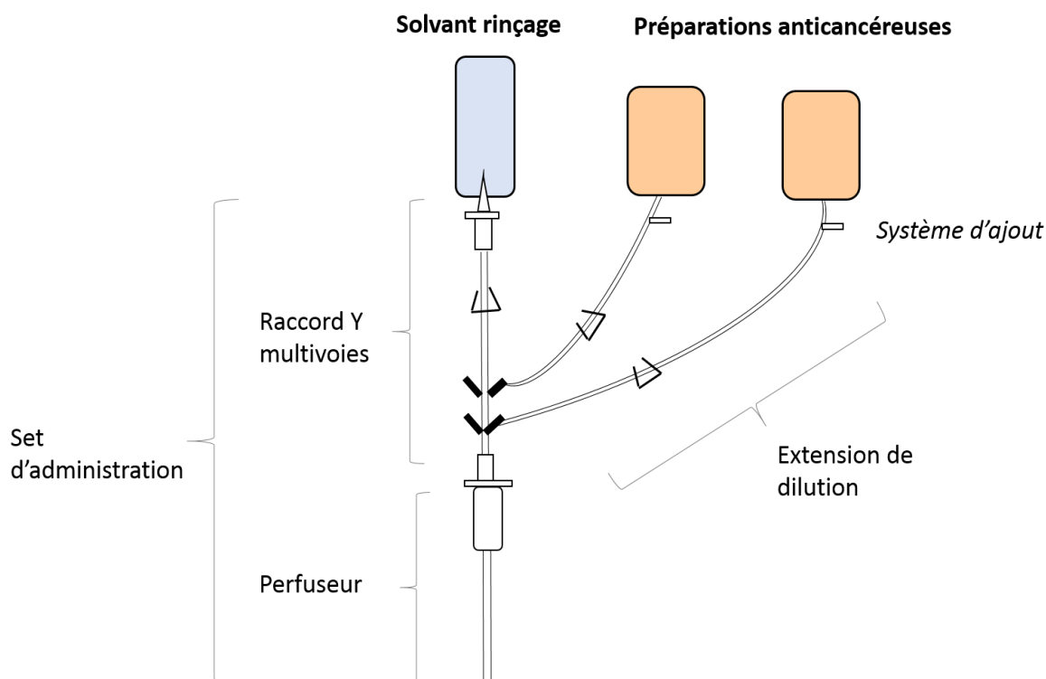
Figure 24 : Arbre à perfusion multiple permettant l'administration sécurisée des anticancéreux
