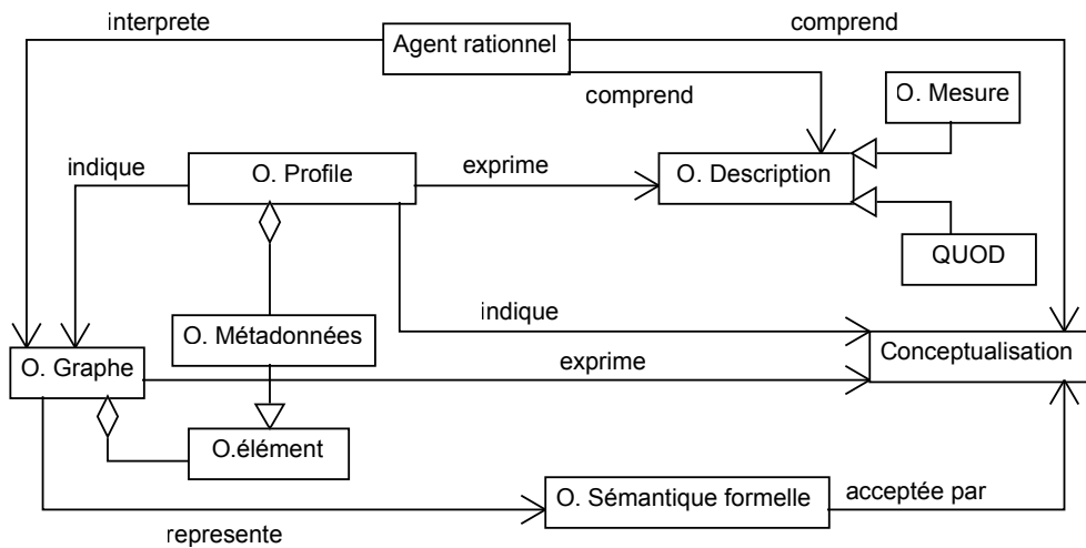
FIGURE 5.1: Diagramme UML (adaptée de Gangemi et al. [49]) illustrant les relations entre les éléments utilisés pour définir une ontologie en tant qu'objet informationnel.
