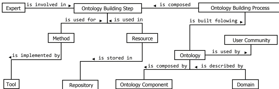
FIGURE 4.2: Les concepts centraux de l'ontologie construite manuellement.
