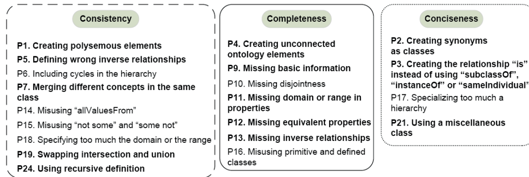
FIGURE A.2: Positionnement de 18 des 24 types d'embûches dans les trois classes d'erreurs de taxonomie (extrait de Poveda et al., 2010 [107]).
