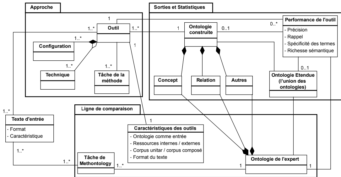
FIGURE 4.1: Diagramme UML résumant les relations entre les éléments utilisés pour notre démarche de comparaison des outils.
