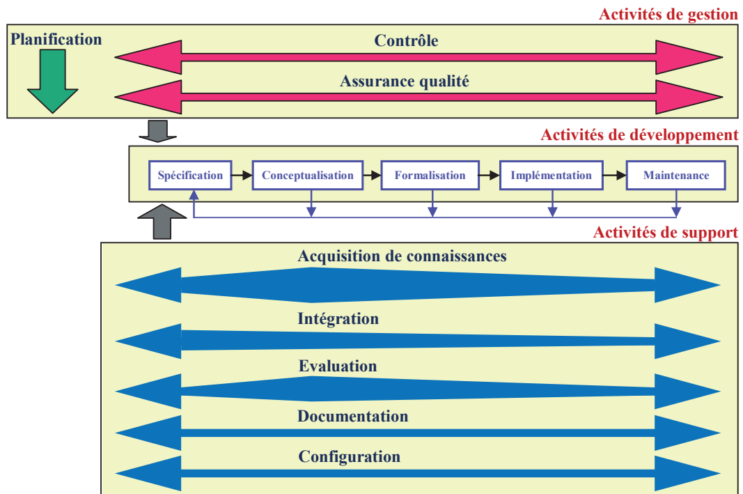
FIGURE 3.2: Les processus de Methontology et les activités qui les composent (image reprise de Gomez-Perez et al., 2001 [55]). Les flèches entre les activités de développement indiquent l'ordre d'exécution des activités et le fait qu'il est toujours possible de revenir à une étape précédente. Les activités de support sont représentées sur forme de flèches allongées : la longueur de la flèche indique la durée de l'activité et son épaisseur indique l'intensité de l'activité (cela permet d'indiquer, par exemple, que l'activité d'acquisition de connaissances connaît la plus forte intensité durant la conceptualisation).
