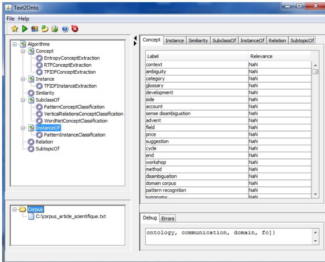
FIGURE 3.10: L'outil associé à l'approche Text2Onto.
