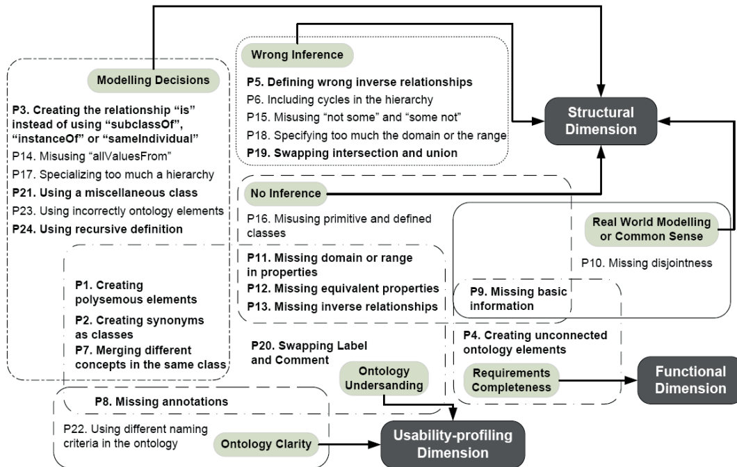
FIGURE A.1: Positionnement des 24 types d'embûches dans les sept classes inspirées des trois dimensions mesurables des ontologies (extrait de Poveda et al., 2010 [107]).
