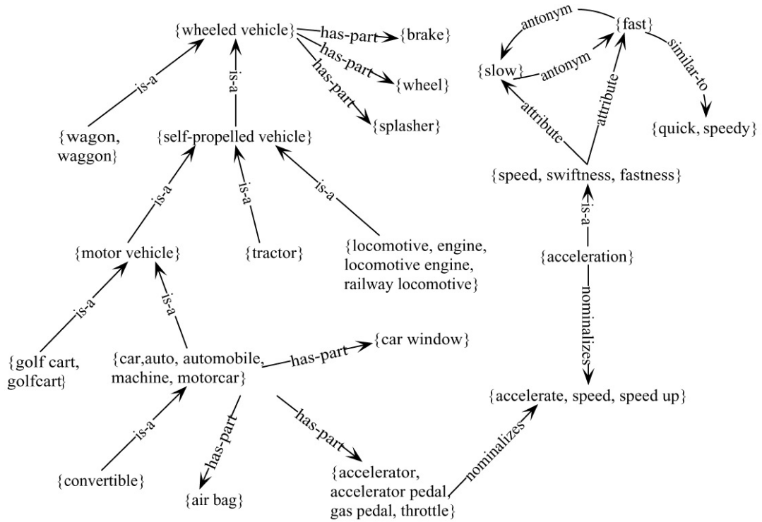
FIGURE 7.1: Illustration des relations sémantiques du synset \{car_n^1, auto_n^1, automobile_n^1, machine_n^6, motorcar_n^1\} associé au mot automobile ; les indices n, v, a indiquent qu'il s'agit d'un nom, d'un verbe ou d'un adjectif; les indices numériques indiquent le numéro du sens du terme avec lequel il est associé au synset; par exemple, machine_n^6 indique que le terme machine est associé au synset avec son sixième sens en tant que nom, alors qu'il a dans WordNet cinq autres sens en tant que nom et deux sens en tant que verbe.
