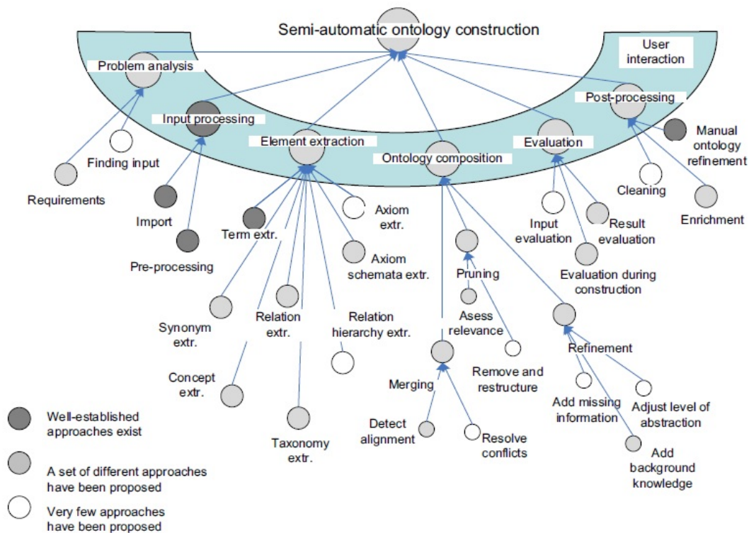
FIGURE 3.8: Les tâches qui composent le processus de construction automatique d'une ontologie. Mise en évidence des tâches pour lesquelles il n'existe aucune approche automatique (image reprise de [13]).
