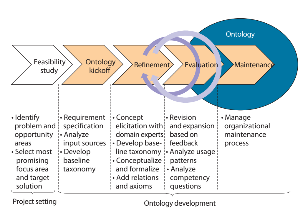
FIGURE 3.4: Les processus de la méthodologie On-To-Knowledge (image reprise de Staab et al., 2001 [123]).
