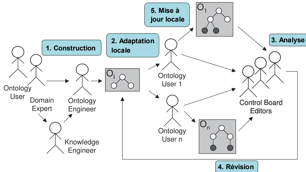
FIGURE 3.5: Les étapes du processus de construction proposé par DILIGENT (image reprise de [103]).
