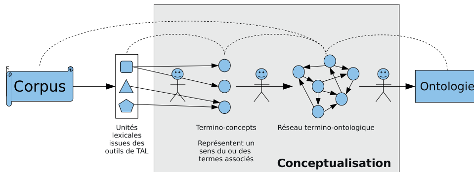
FIGURE 3.9: Les étapes du processus de construction d'une ontologie proposé par Terminae (image reprise de [87]).
