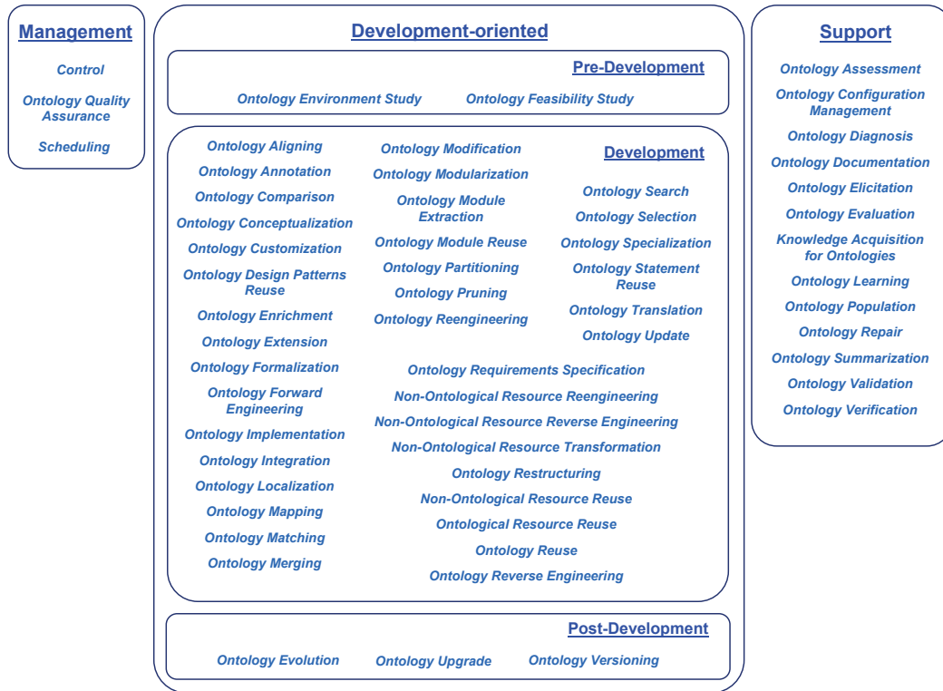
FIGURE 3.6: Classification des 59 activités qui peuvent faire partie du processus de développement d'une ontologie proposé par NeOn (image reprise de [127]).
