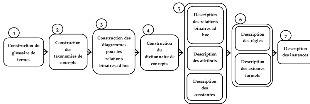
FIGURE 3.3: Les tâches qui composent l'activité de conceptualisation de Methontology (figure adaptée de Gomez-Perez et al., 2001 [55]).
