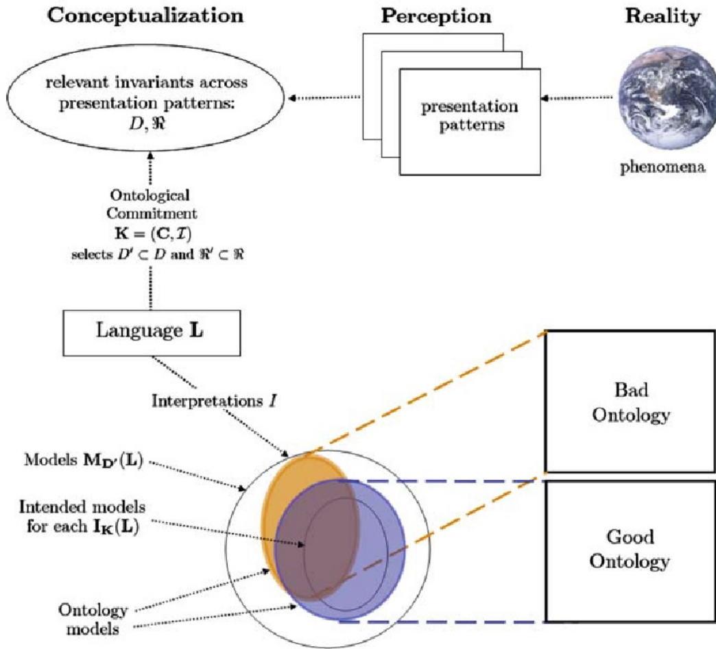
FIGURE 2.3: Illustration des relations entre une conceptualisation, le langage utilisé pour sa formalisation, les modèles intentionnels et l'ontologie (extrait de Guarino et al. (2009) [60]).
