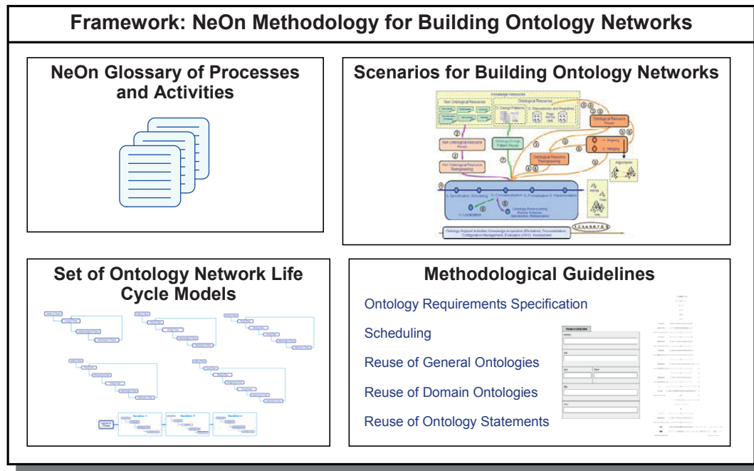
FIGURE 3.7: Vue globale des principaux points forts de la méthodologie NeOn (image reprise de [127]).
