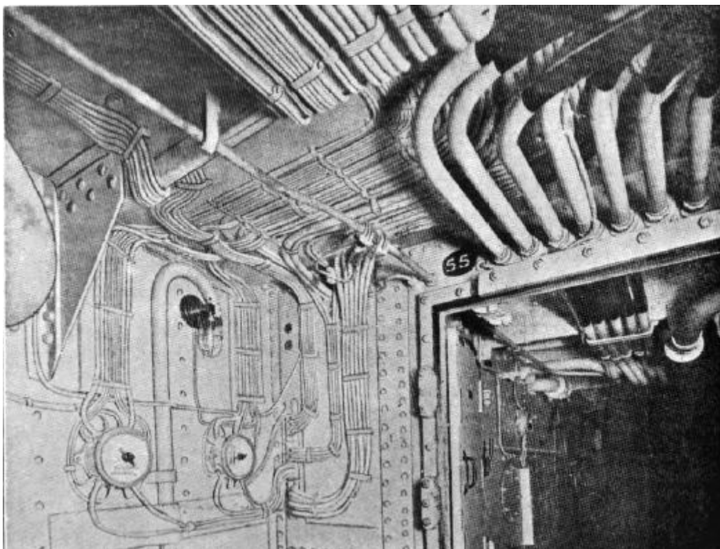
Illustration 77 : Passage de cloison étanche avec un disque plat
