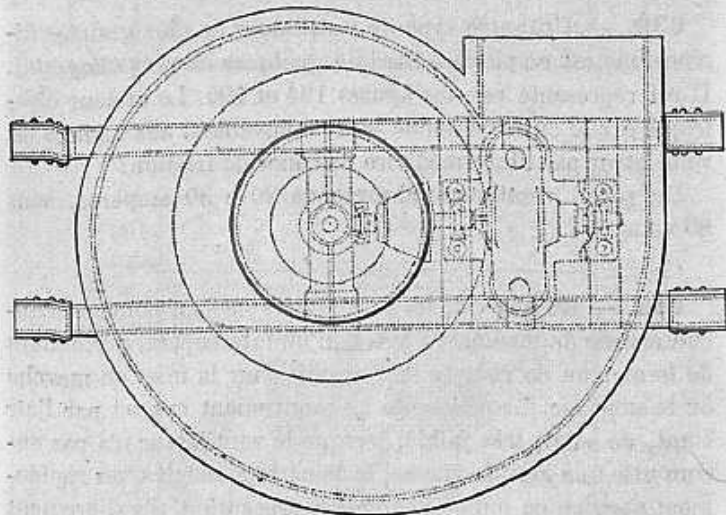
Fig. 195. — Ventilateur de refoulement. Plan; échelle \frac{1}{20} .
