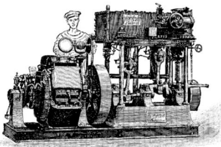
Illustration 33 : Générateur d'électricité du cuirassé l'Indomptable.
