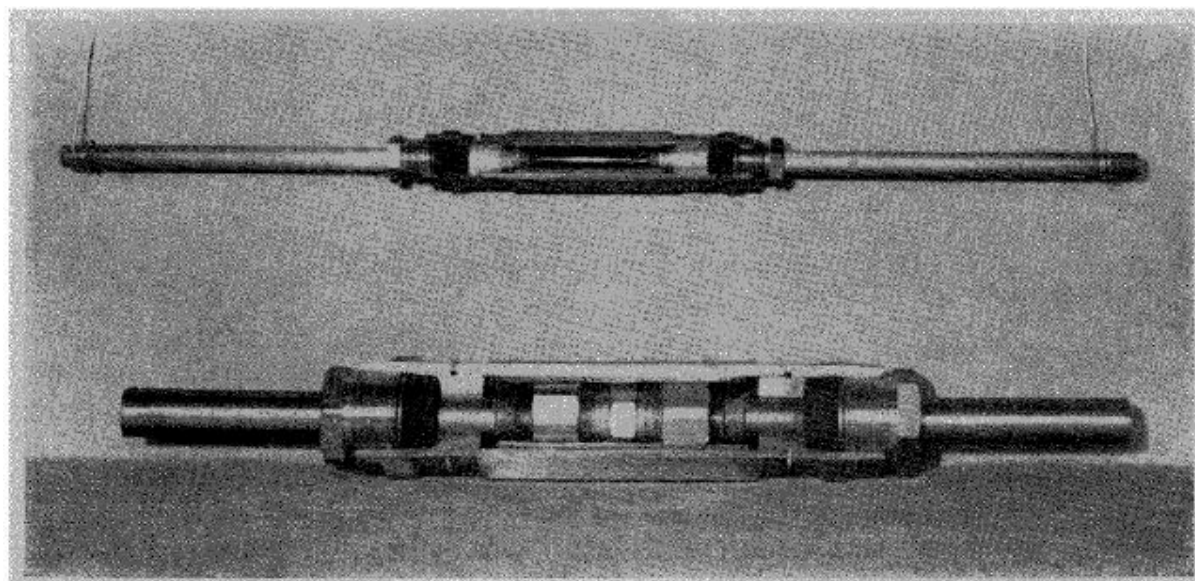
Fig. 4. — CÂBLE PYROTÉNAX : Joints à clanches.
