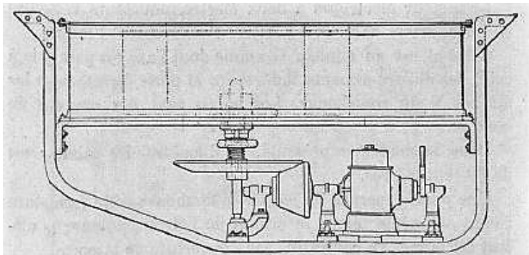
Fig. 194. — Ventilateur de refoulement. Élévation; échelle \frac{1}{20} .
