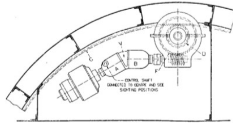
Fig. 12. — Appareil Williams et Janney A V B commandant la rotation d'une tourelle de cuirassée par la transmission hélicoïdale F D C. On doit pouvoir obtenir, pour satisfaire à certaines conditions du pointage des canons de la turbine, réduire de 2 000 fois en C la vitesse de A et de sa dynamo.
