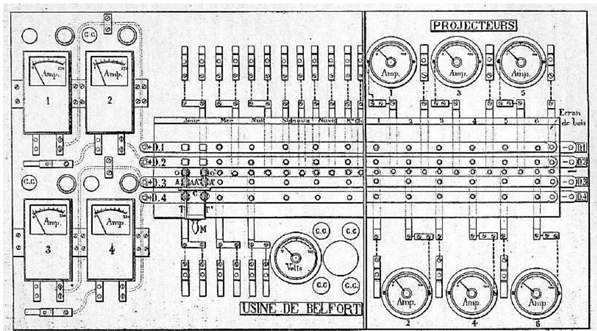
Illustration 62 : Tableau type 1890
