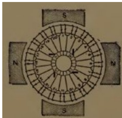
Illustration 151 : Rotor avec 2 collecteurs
