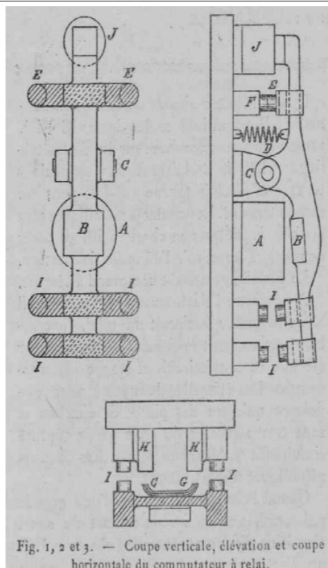
Illustration 113 : Relais à 3 contacts
