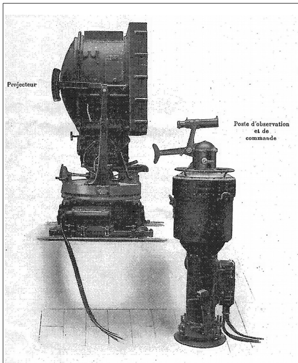
Fig. 5. — Projecteur de 90 c/m. de diamètre, type cuirassé et croiseur.
