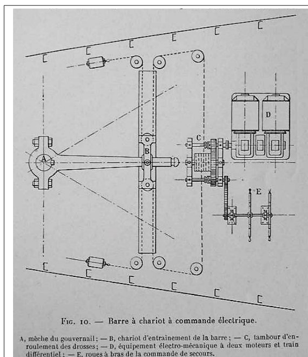
Illustration 41 : Commande électrique du gouvernail
