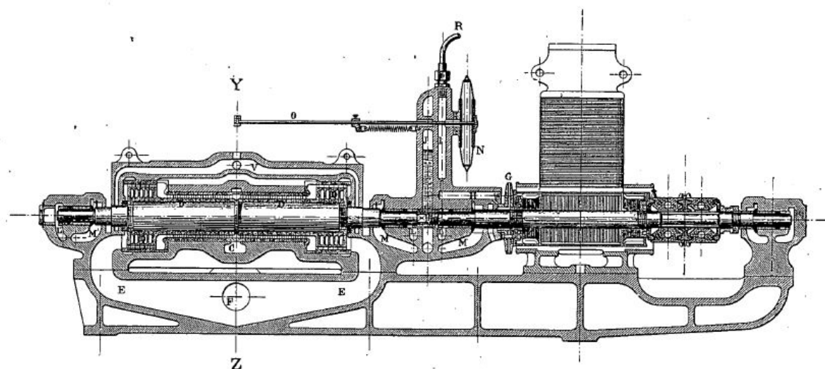
Illustration 142 : Turbo-dynamo SAUTTER-LEMONNIER
