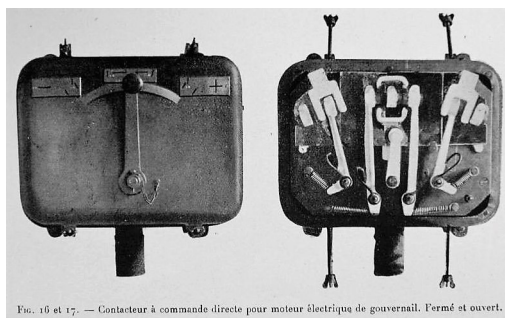
Fig. 16 et 17. — Contacteur à commande directe pour moteur électrique de gouvernail. Fermé et ouvert.
