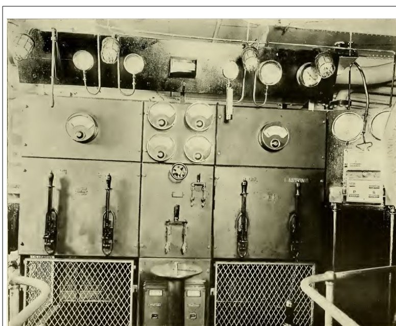
Illustration 75 : Tableau de distribution principal de l'USS Jupiter
