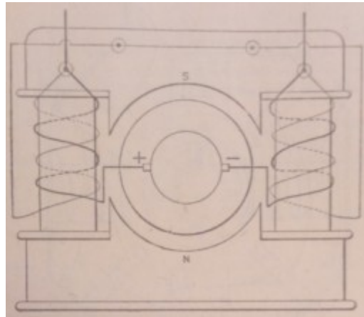
Illustration 145 : Dynamo type H
