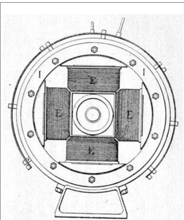
Illustration 147 :Dynamo multipolaire
