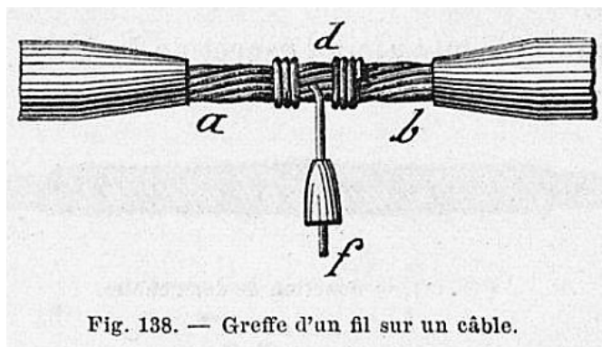
Illustration 57 : Greffe de fil sur un câble
