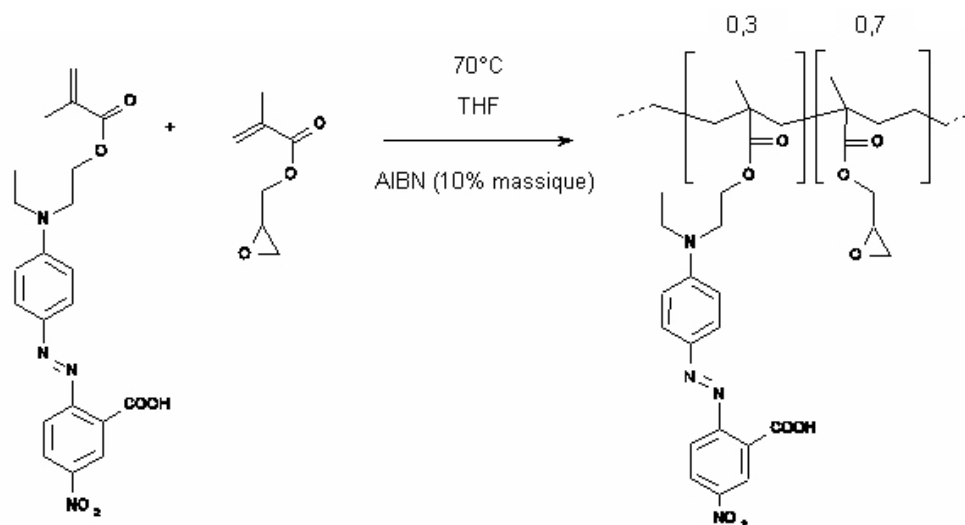
FIG. 3.4 – Étape de polymérisation du PIH/PII
