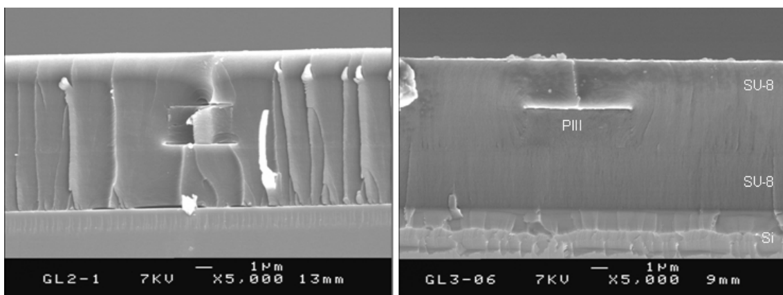
FIG. 4.13 – Images MEB de guides d'onde en polymère PIII entouré de gaines SU-8 sur substrat de silicium, les motifs de guides présentent une hauteur de 2,5\text{ }\mu\text{m} pour une largeur de 4\text{ }\mu\text{m} et 6\text{ }\mu\text{m} respective sur l'image de gauche et de droite
