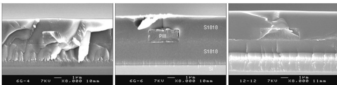
FIG. 4.12 – Images MEB de guides en polymère PIII entourés de gaines S1818 sur substrat de silicium, les motifs de guides présentent une hauteur de 1,7\text{ }\mu\text{m} pour une largeur de 2, 4 et 6\text{ }\mu\text{m} respectivement de gauche à droite
