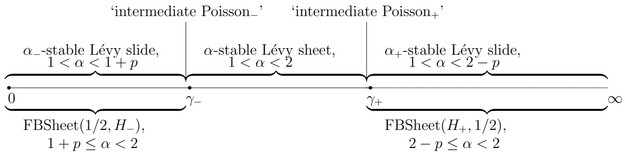
Figure: V_\gamma en fonction de \gamma variant de 0 à \infty , 1 < \alpha < 2 , 0 < p < 1 .
