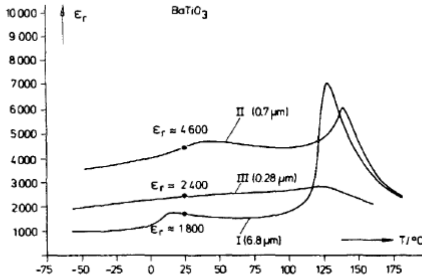
Figure 1.21 : Evolution de la permittivité en fonction de température de \text{BaTiO}_3 pour différentes tailles de particules [62]
