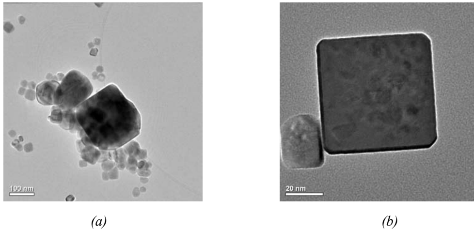
Figure 2.21 : Image MET de particules de a) BTO et b) STO après traitement acide.
