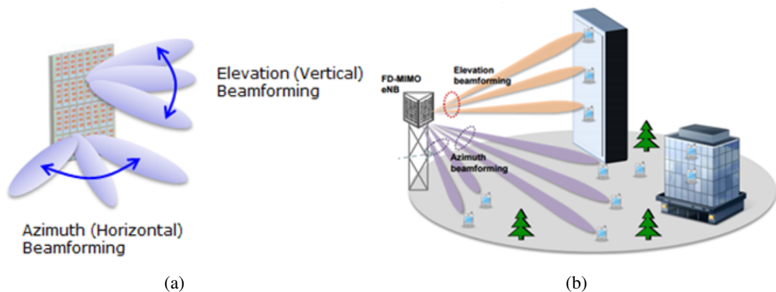
FIGURE 1.15 : Couvertures radioélectriques dans le cas de la FD MIMO
