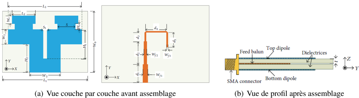
FIGURE 2.10 : Structure de l'antenne dipôle triplaque améliorée [50]
