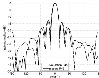
(b) 2,2 GHz P45
