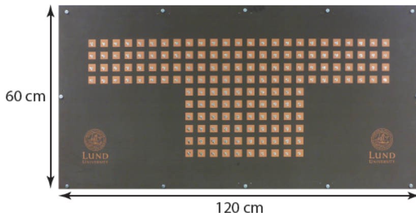
FIGURE 1.17 : Antenne de test du Massive MIMO
