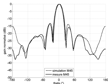
(d) 1,7 GHz M45
