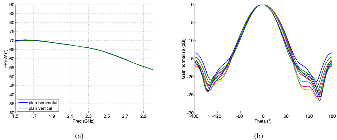
FIGURE 2.21 : Ouvertures plan horizontal et vertical (a) et diagrammes de rayonnement associés (b) à l'antenne Kathrein
