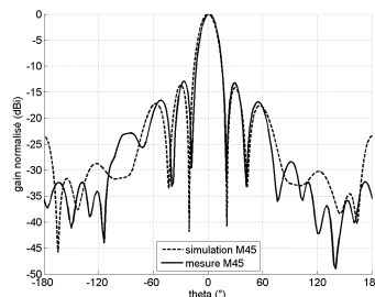
(e) 2,2 GHz M45
