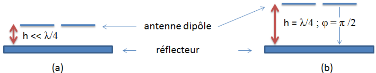
FIGURE 2.23 : Principe d'interférences destructrices (a) ou constructives (b) en fonction de la position du réflecteur métallique
