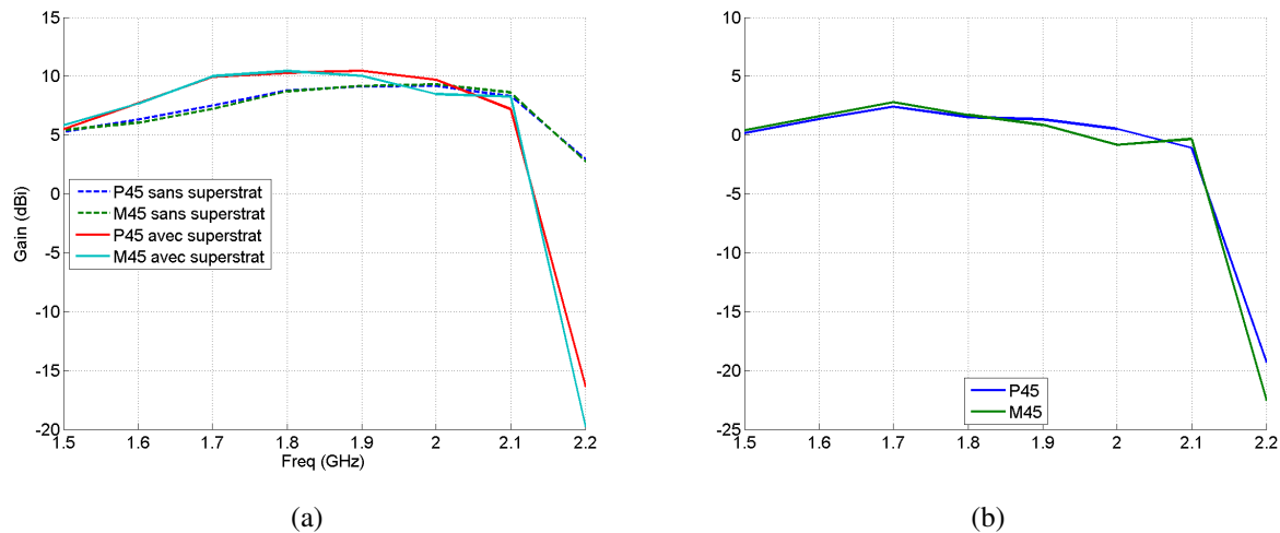
FIGURE 2.46 : Gains simulés sur les deux polarisations de Powerwave avec et sans le superstrat homogène (a) et différence de gain entre les deux configurations sur les deux polarisations (b)
