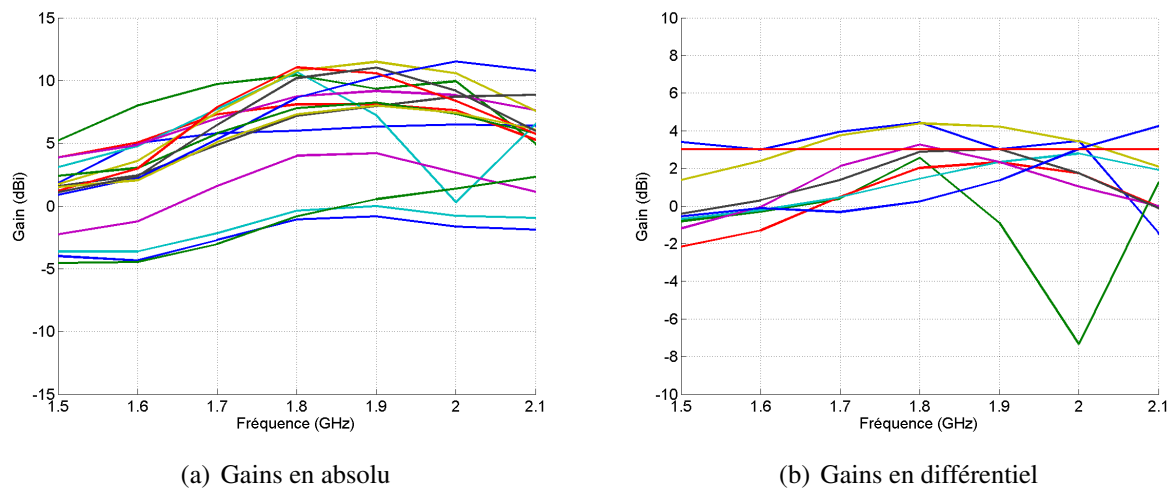
FIGURE 2.48 : Résultats de l'étude des différents cas résumés dans le tableau 2.9 en absolu (a) et en différentiel par rapport à l'antenne Powerwave complète (b)
