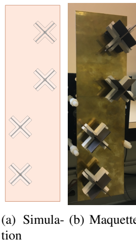
FIGURE 4.33 : Principe de l'antenne réseau avec symétrie centrale des éléments rayonnants unitaires en simulation (a) et en maquette (b)
