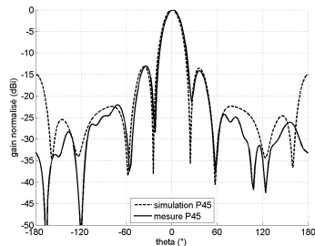
(a) 1,7 GHz P45
