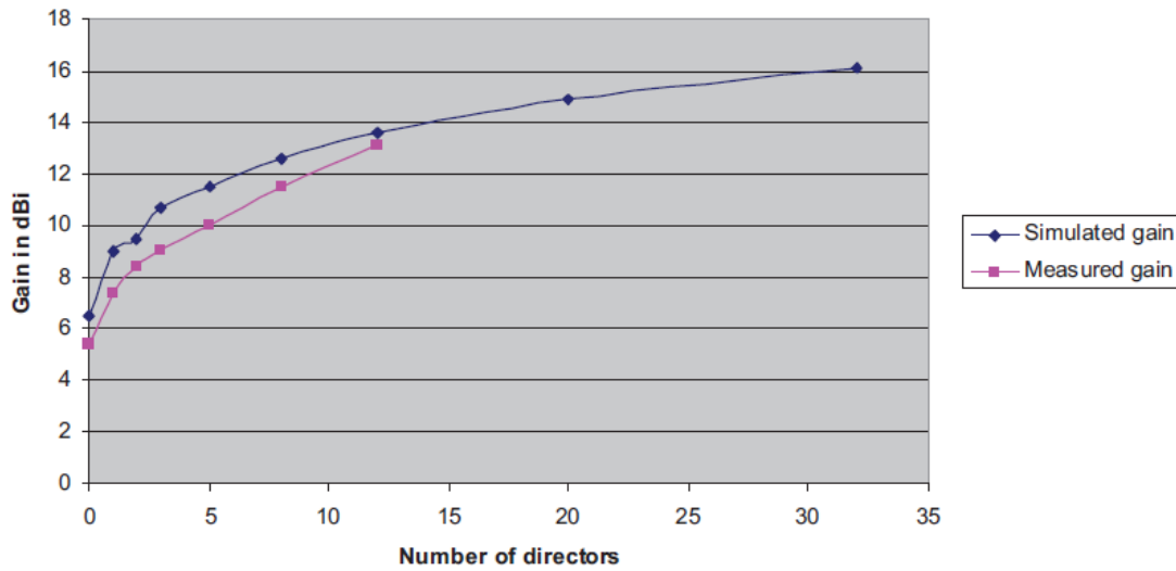
FIGURE 3.14 : Détermination du gain en fonction du nombre de directeurs sur une antenne Yagi [88]
