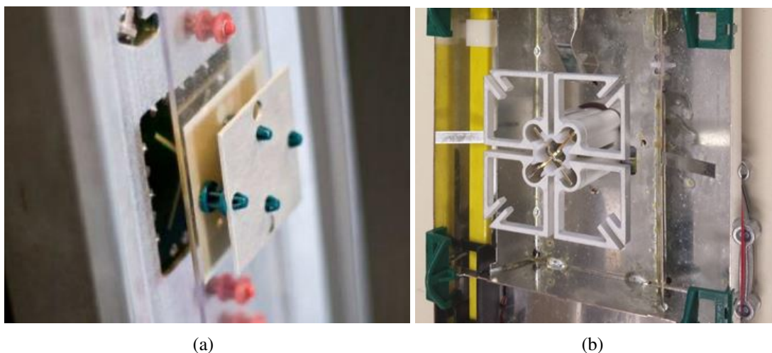
FIGURE 2.13 : Éléments rayonnants Powerwave (a) et Kathrein (b)
