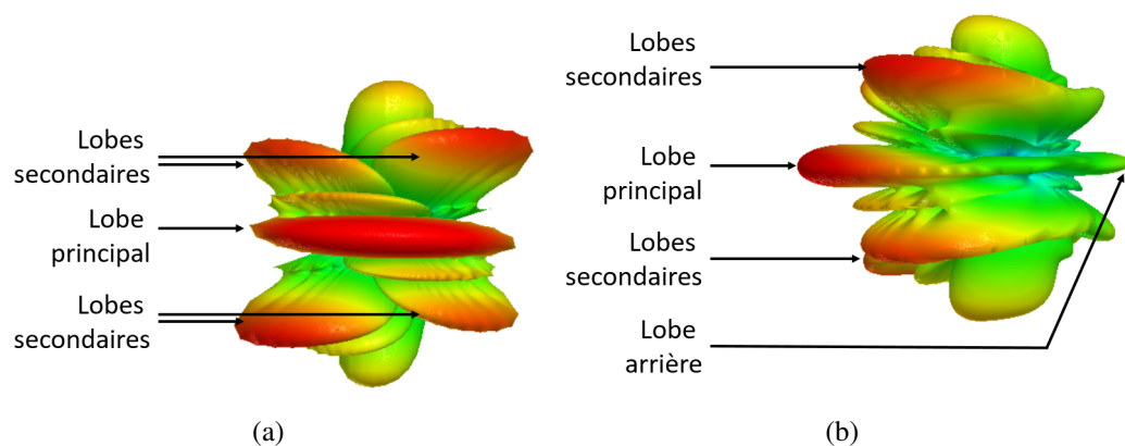
FIGURE 4.31 : Diagramme de rayonnement vu de face (a) et de profil (b) de l'antenne réseau alternée à six éléments unitaires
