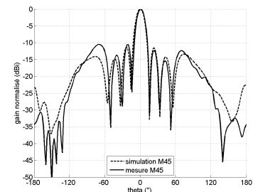
(f) 2,7 GHz M45
