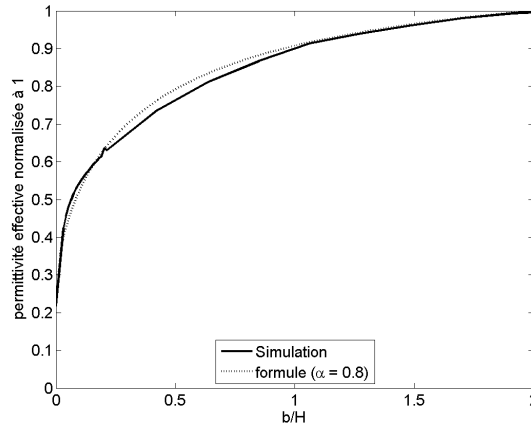
FIGURE 3.3 : Evolution de la permittivité effective représentée par la formule 3.3 normalisée et comparée par la simulation HFSS
