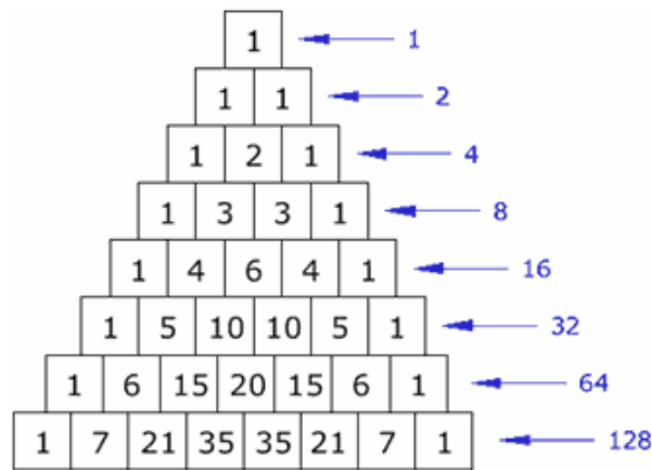
FIGURE 4.8 : Tableau de Pascal issu de la formule 4.3 calculant les pondérations à appliquer pour un réseau binomial
