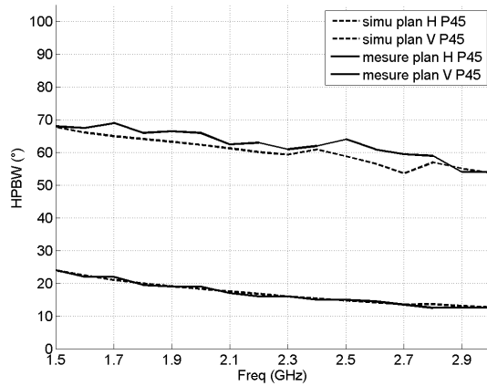
(a) Polarisation P45
