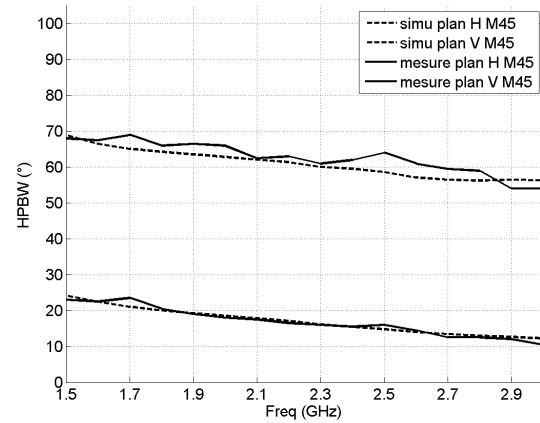
(b) Polarisation M45
