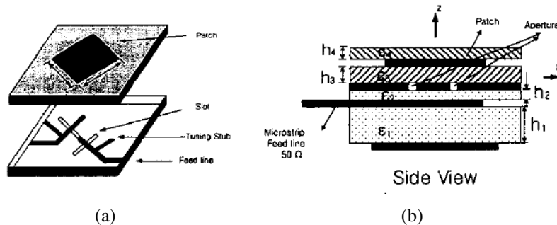
FIGURE 2.2 : Structure à fente rectangulaire et un patch [40]
