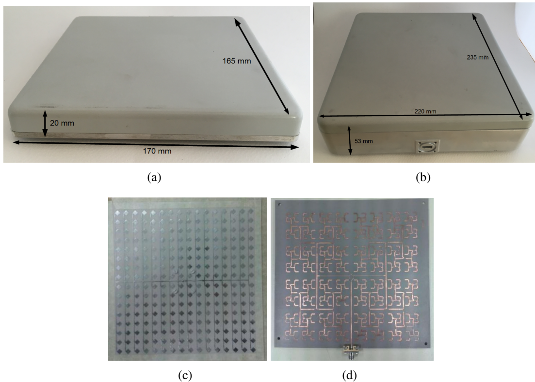
FIGURE 1.29 : Antennes plates FH version 1 boîtier (a) et circuit antenne (c) et classe 3 boîtier (b) et circuit d'alimentation (d)
