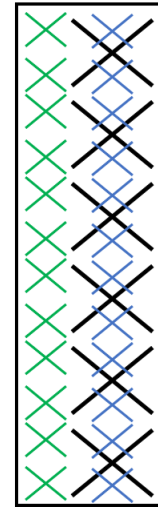
FIGURE 4.43 : Zoom sur les éléments rayonnants de l'antenne Huawei AQU4518R0 à gauche et sa reprise schématique à droite (b)
