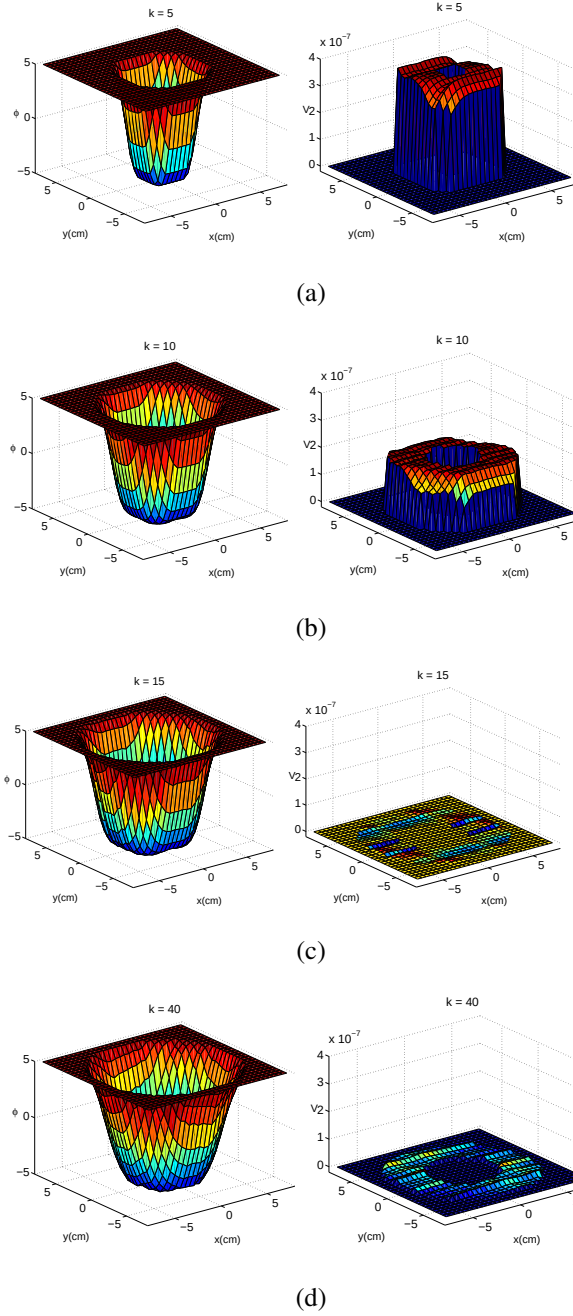
Figure 3.9: Evolution de la fonction de niveau \phi (gauche) et de la vitesse V (droite), dans la tranche S_m à z = 0 , avec la méthode «bande étroite» dans le cas 'ortho+1arb' aux itérations : (a) k = 5 ; (b) k = 10 ; (c) k = 15 ; (d) k_{final} = 40 .
