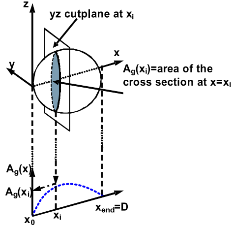
Figure 2.2: Illustration de la fonction de profil géométrique d'un objet, A_g(x) , selon la direction x . D est la dimension caractéristique de l'objet dans la direction x .
