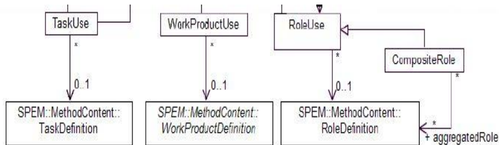
Figure 5.12 – Quelques associations SPEM exploitées pour gérer les correspondances entre les connaissances PLs [92].
