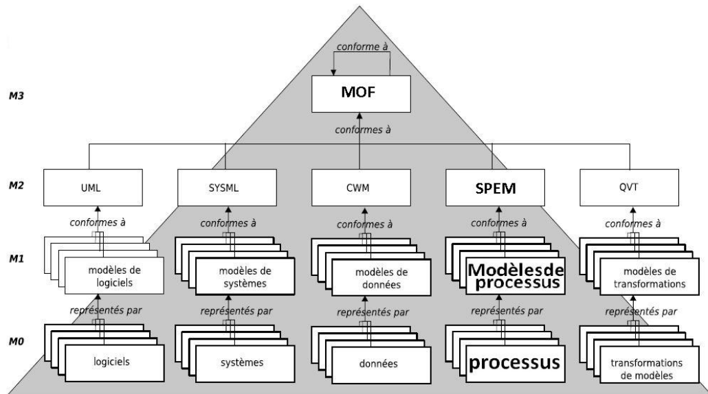
Figure 1.2 – L'architecture à 4 niveaux de l'OMG [35].
