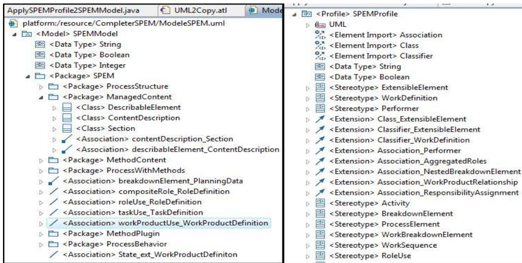
Figure 5.5 – Les modèles sources du module ApplySPEMProfil2SPEMModel décrit en UML.
