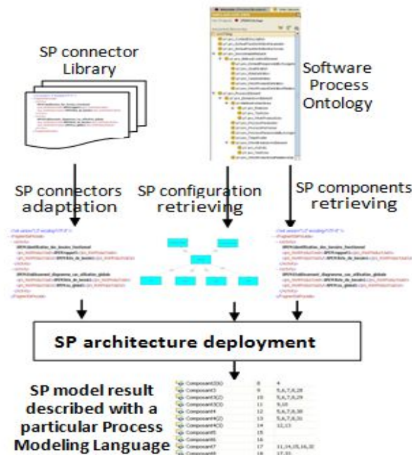
Figure 4.13 – Les étapes de l'ingénierie par la réutilisation des PLs.
