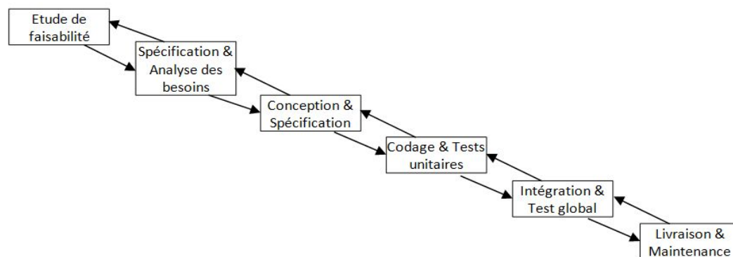
Figure 1.1 – Cycle de vie du logiciel Waterfall (Royce 1970) [110].
