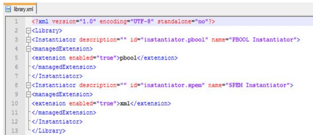
Figure 5.13 – Librairie qui permet de sauvegarder les informations des instanciateurs.
